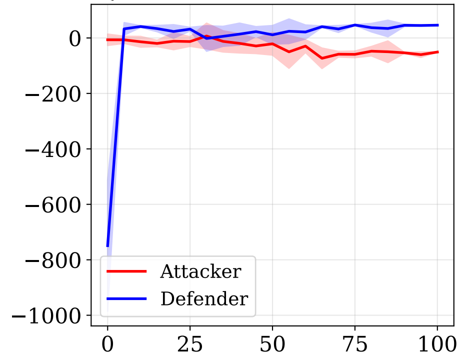
DQN Att vs PPO Def: Reward
